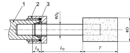
Рис. 1: Длина зажима зажимного патрона и цангового зажима
