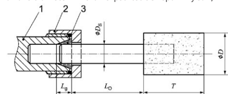
Fig. 1: Inspänningslängd från spännchuck och spännhylsa
