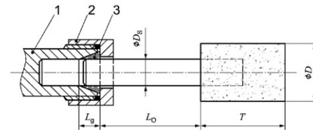
Bild 1: Einspannlänge von Spannfutter und Spannzange
