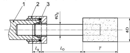
Фиг. 1: Дълбочина на захвата на патронника и на цангата
