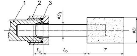
Resim 1: Germe aynası ile germe pensi arasındaki gerdirmeye uzunluğu
