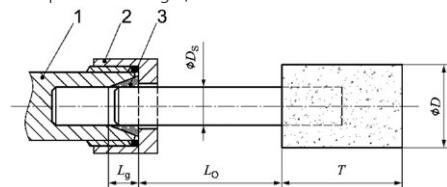
Figure 1: Longueur de serrage du mandrin et de la pince de serrage Légende
