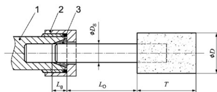
Figur 1: Kjoksens og festemekanisms spennlengde
