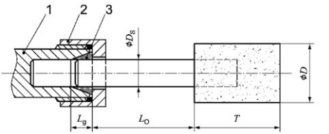
Εικόνα 1: Μήκος τοποθέτησης εργαλείου-κόλτε και κόλτε
