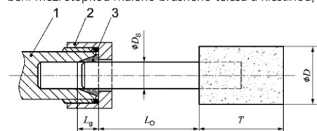
Obrázek 1: Délka upnutí sklíďidla a kleštiny
